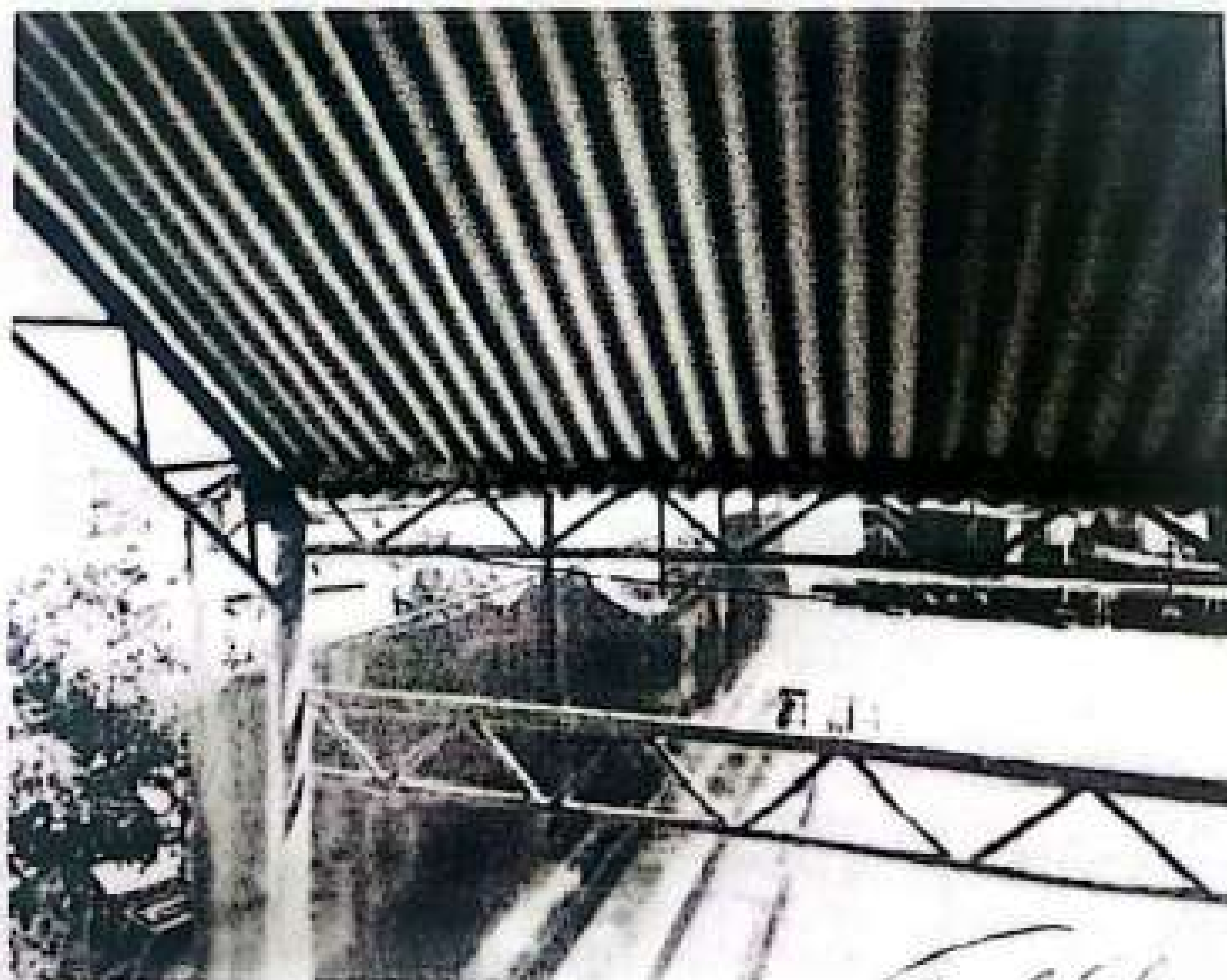
Fotografía 2: Se observa que en los anclajes y vigas de distribución del coliseo de nivel primaria, presenta corrosión y deterioro de sección.
